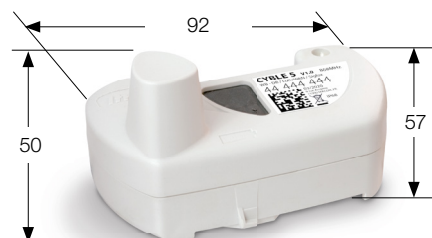
Dimensioner (mm)
